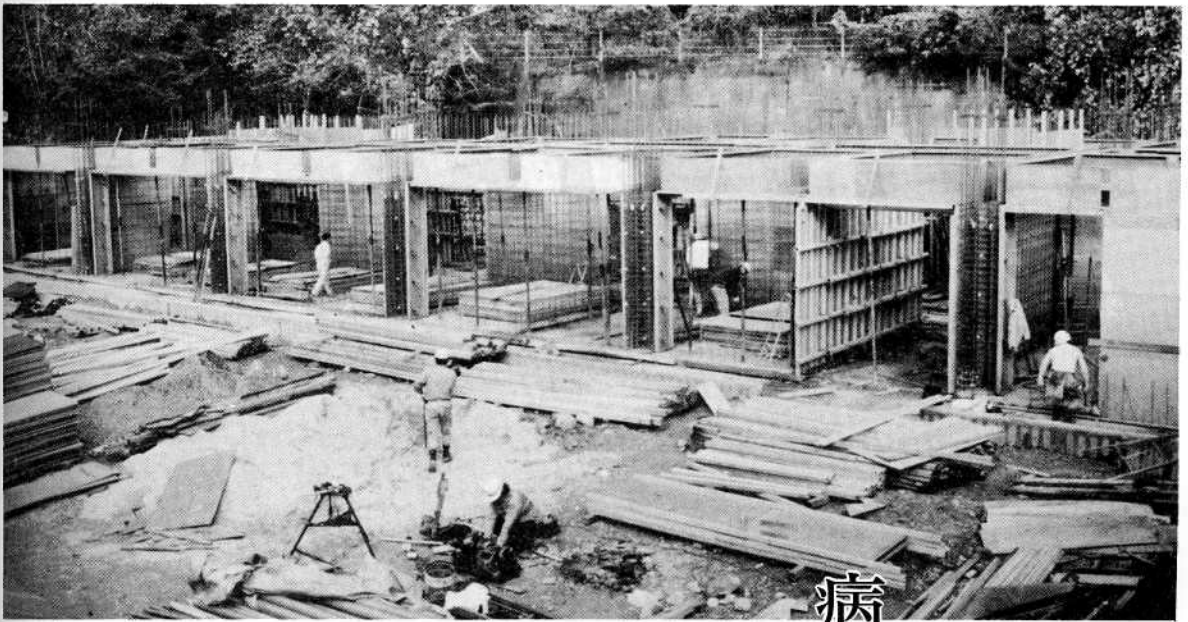
基礎工事が終わり、1階の型枠工事が進められている病院棟
